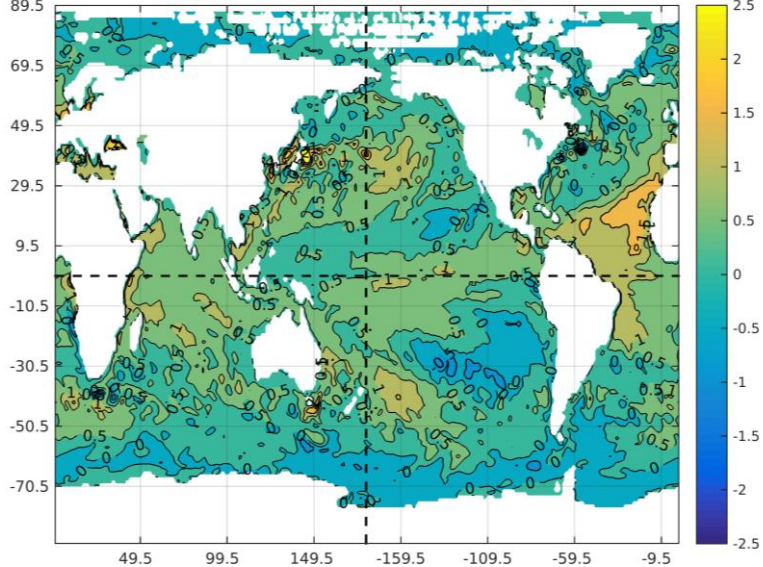
SST MAM IC:Mar2024
