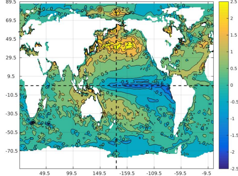
SST ASO IC:Mar2024
