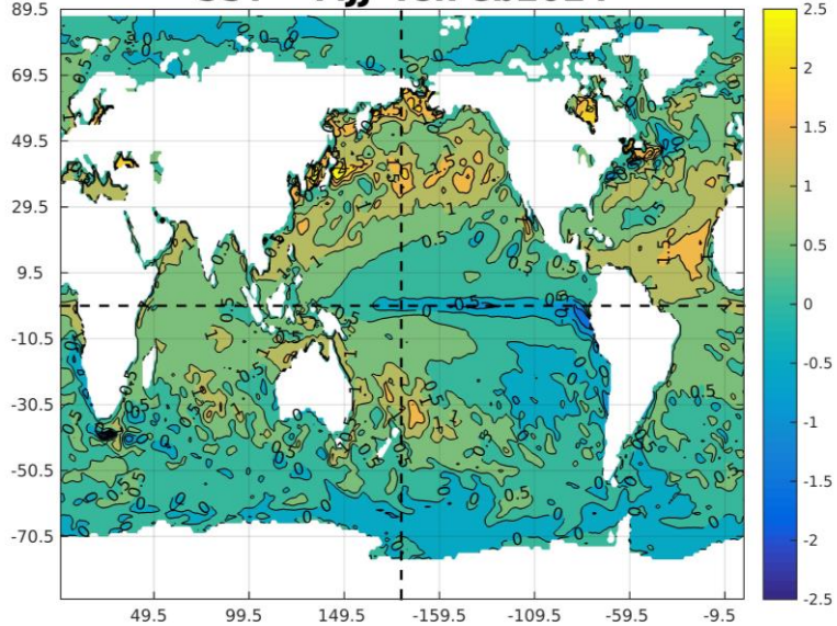
SST MJJ IC:Feb2024
