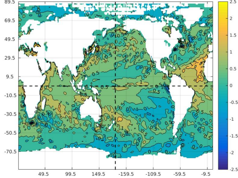
SST MAM IC:Feb2024
