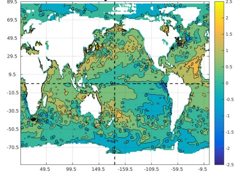
SST AMJ IC:Feb2024
