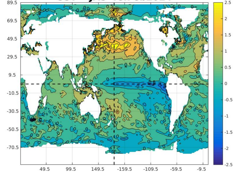
SST JAS IC:Feb2024
