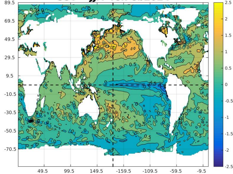
SST JJA IC:Feb2024
