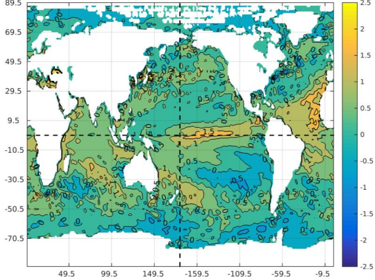
SST FMA IC:Feb2024
