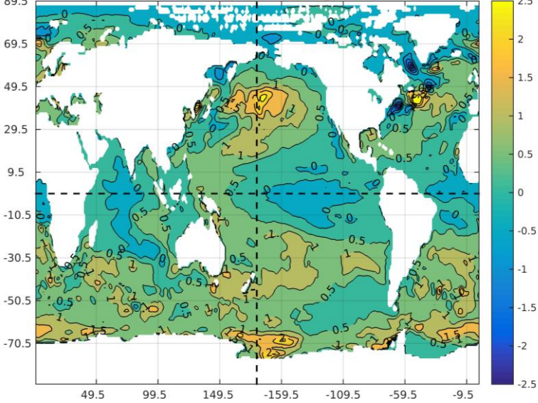
SST NDJ IC:Aug2025
