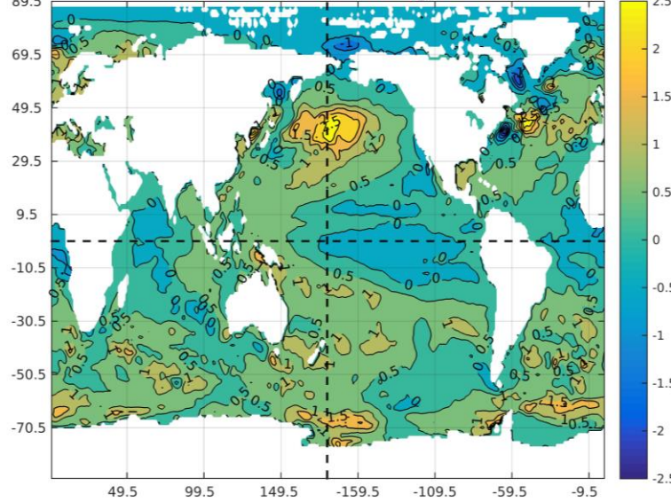
SST OND IC:Aug2025
