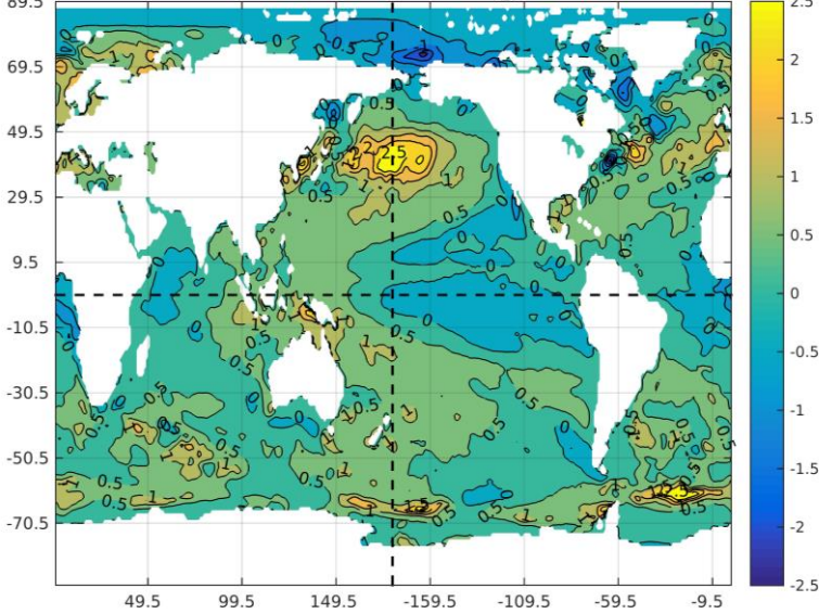
SST SON IC:Aug2025
