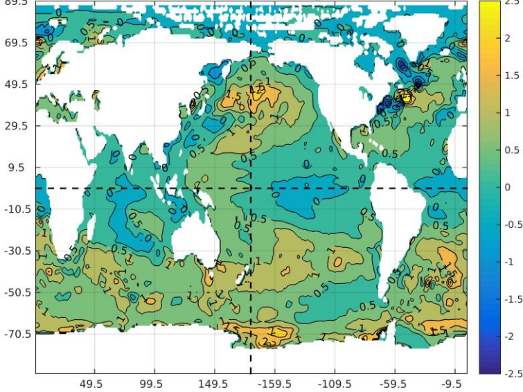
SST DJF IC:Aug2025
