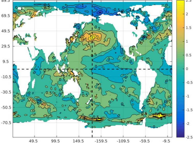
SST ASO IC:Aug2025
