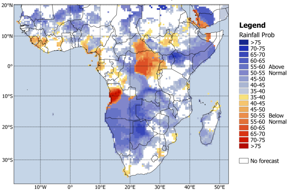
MAM 2025 Rainfall; ICs: Jan
