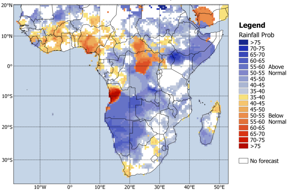
MAM 2025 Rainfall; ICs: Dec
