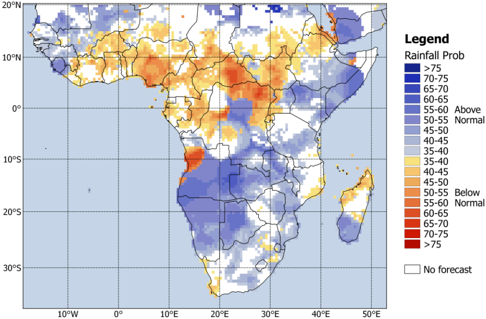
MAM 2025 Rainfall; ICs: Feb
