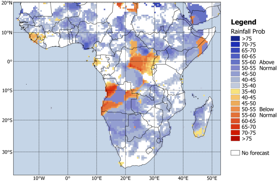
MAM 2025 Rainfall; ICs: Mar
