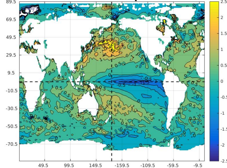
SST SON IC:Apr2024
