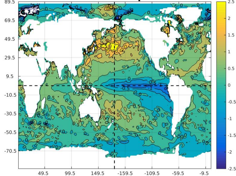
SST ASO IC:Apr2024
